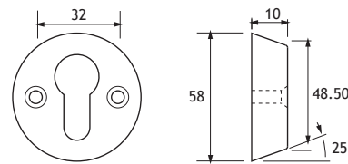
PR4-58E Euro Profile Escutcheon
