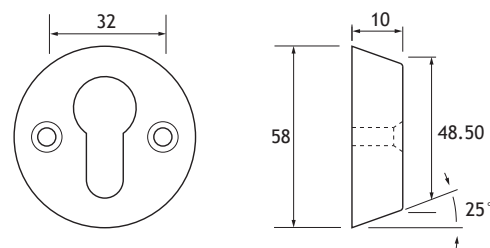
PR4-58E Euro Profile Escutcheon
