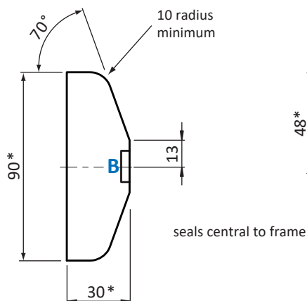
Hanging Jamb
